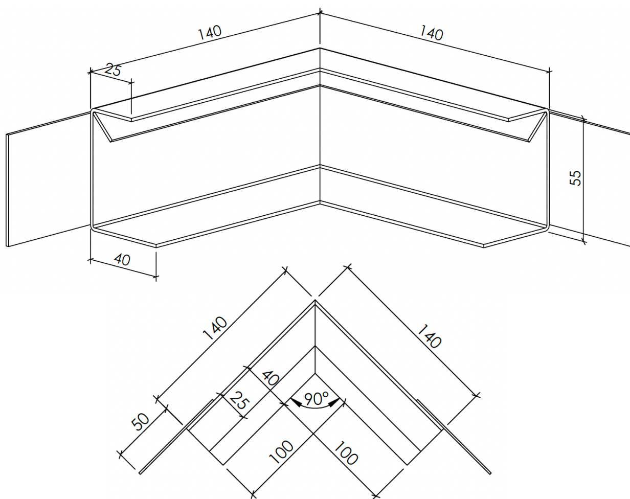
BOVENAANZICHT
