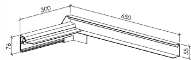
Basisprofiel
