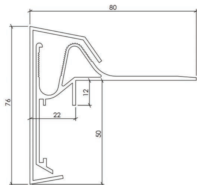
Basisprofiel
