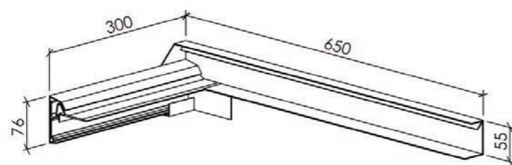
Basisprofiel
