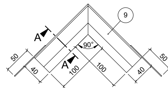
bovenaanzicht
